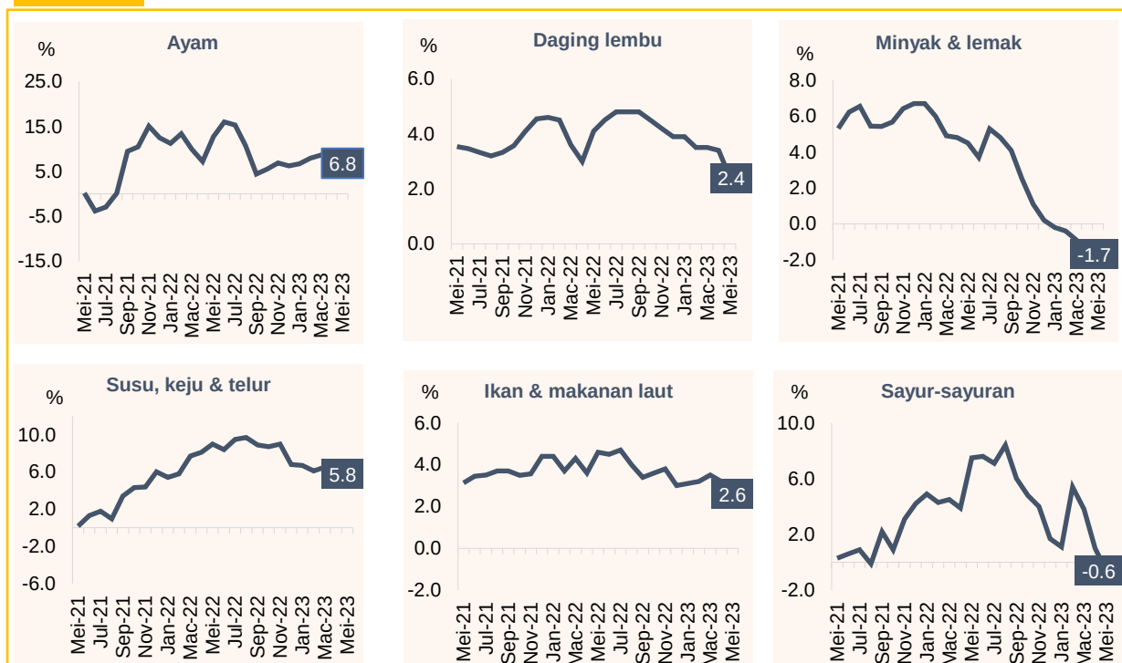
Carta 11 Inflasi Makanan Terpilih bagi Kumpulan Pendapatan Bawah RM3,000, Mei 2021 – Mei 2023
