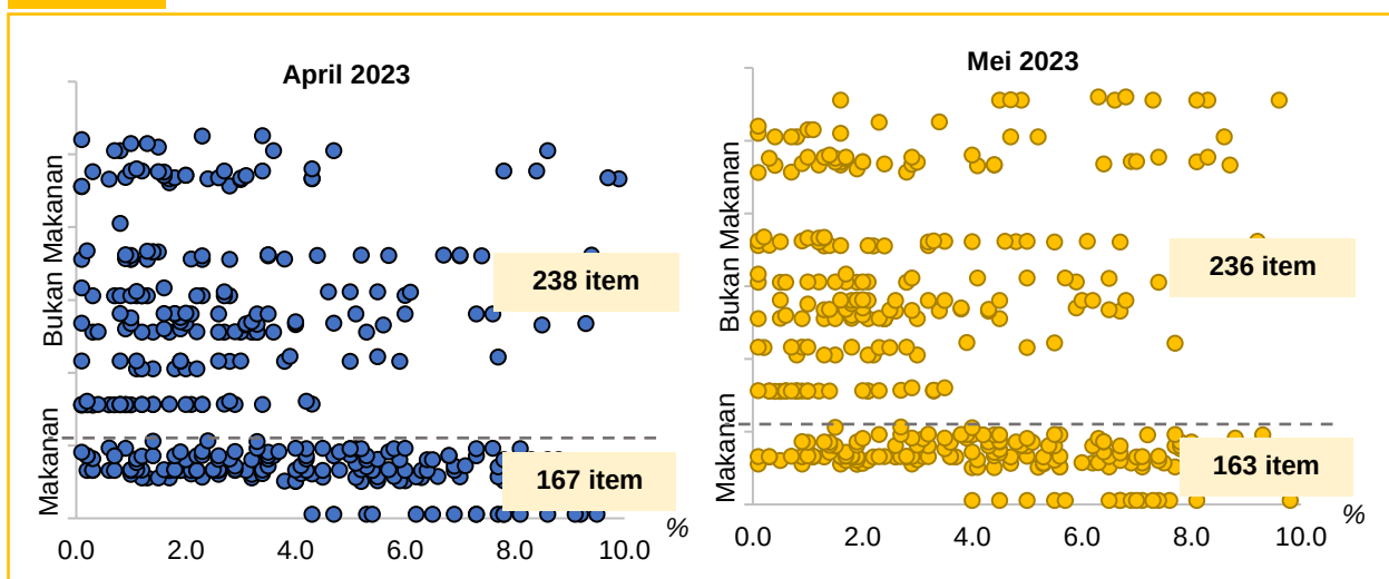
Carta 6 Taburan Inflasi Makanan dan Bukan Makanan yang Meningkat \leq 10\% , April 2023 & Mei 2023
