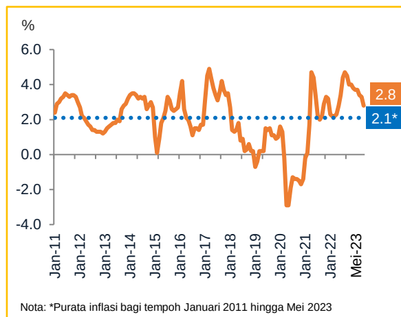
Carta 2 Inflasi Keseluruhan Malaysia, Januari 2011 – Mei 2023
