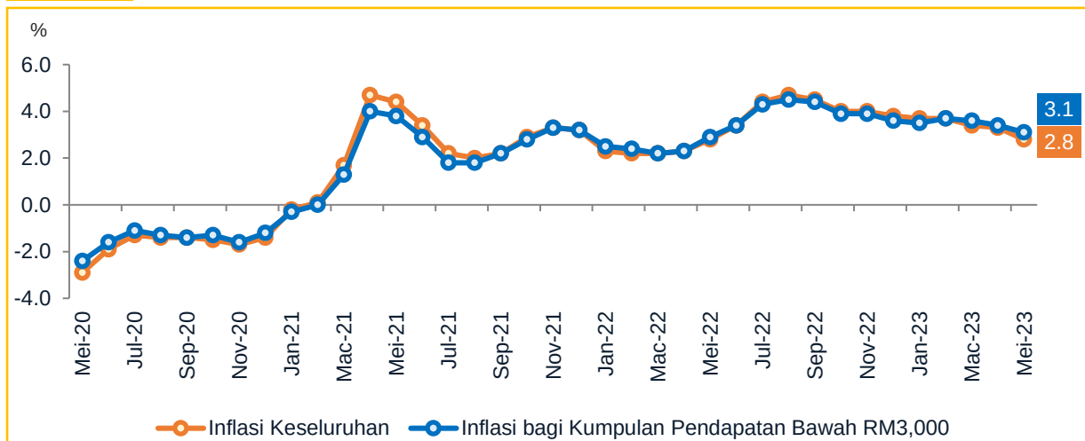
Carta 10 Inflasi bagi Kumpulan Pendapatan Bawah RM3,000, Mei 2020 – Mei 2023
