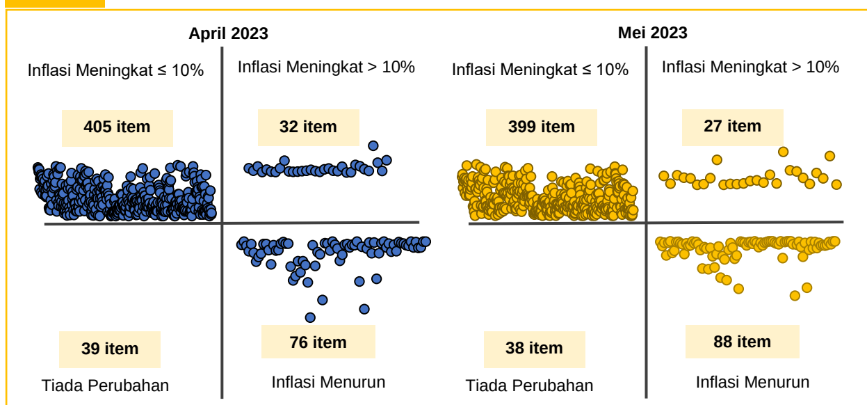
Carta 5 Inflasi mengikut Kuadran, April 2023 & Mei 2023
