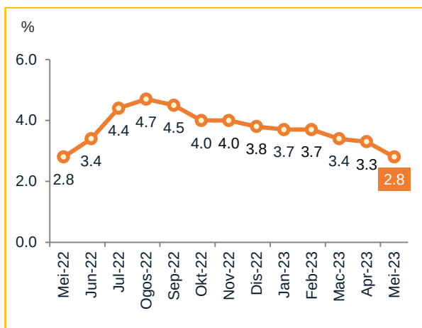
Carta 1 Inflasi Keseluruhan Malaysia, Mei 2022 – Mei 2023
