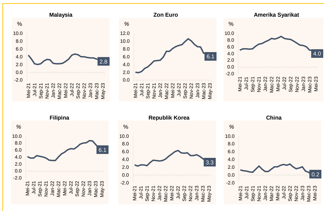
Carta 12 Inflasi bagi Negara Terpilih, Mei 2021 – Mei 2023
