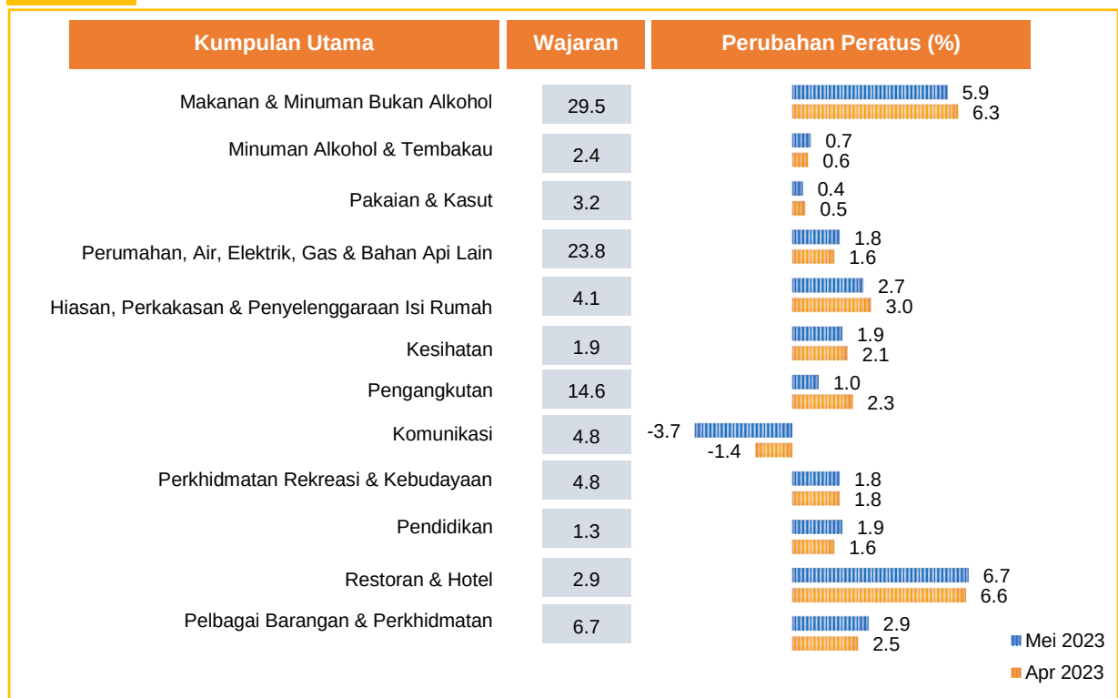
Carta 3 Inflasi mengikut Kumpulan Utama, April 2023 & Mei 2023
