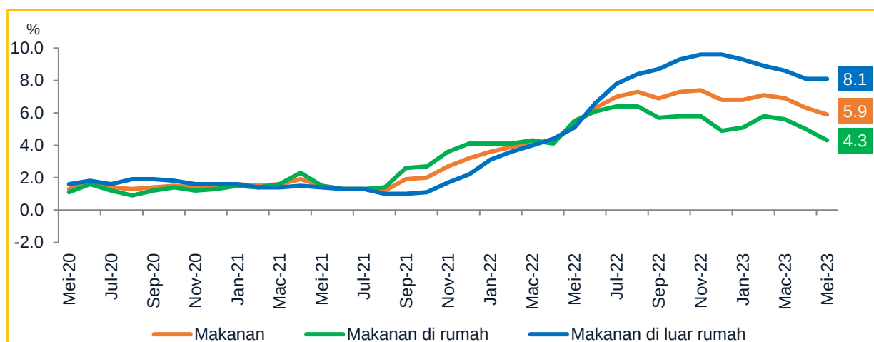
Carta 7 Inflasi bagi Makanan & Minuman Bukan Alkohol, Mei 2020 – Mei 2023
